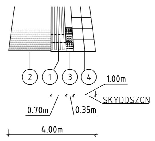
TYPSNITT, PERRONG SNITT A-A, SKALA 1:100
