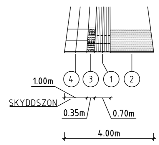
TYPSNITT, PERRONG SNITT B-B, SKALA 1:100
